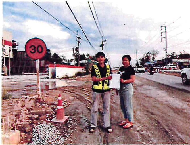
รูปที่ 1 ถนนของโครงการ กม.ที่ 3+354 ด้านซ้ายทาง
